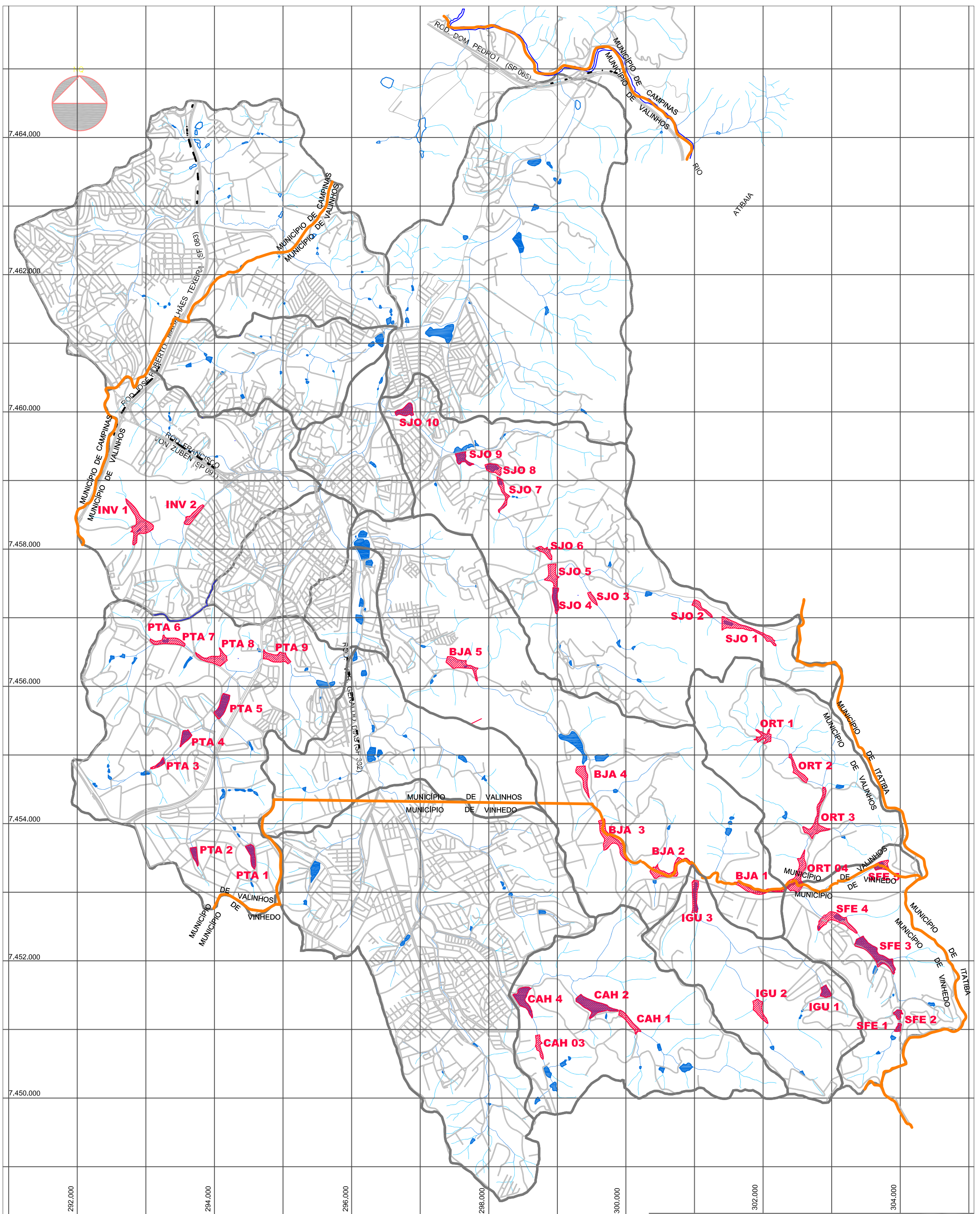
Figura 11 BACIAS DE DETENÇÃO PROJETADAS
